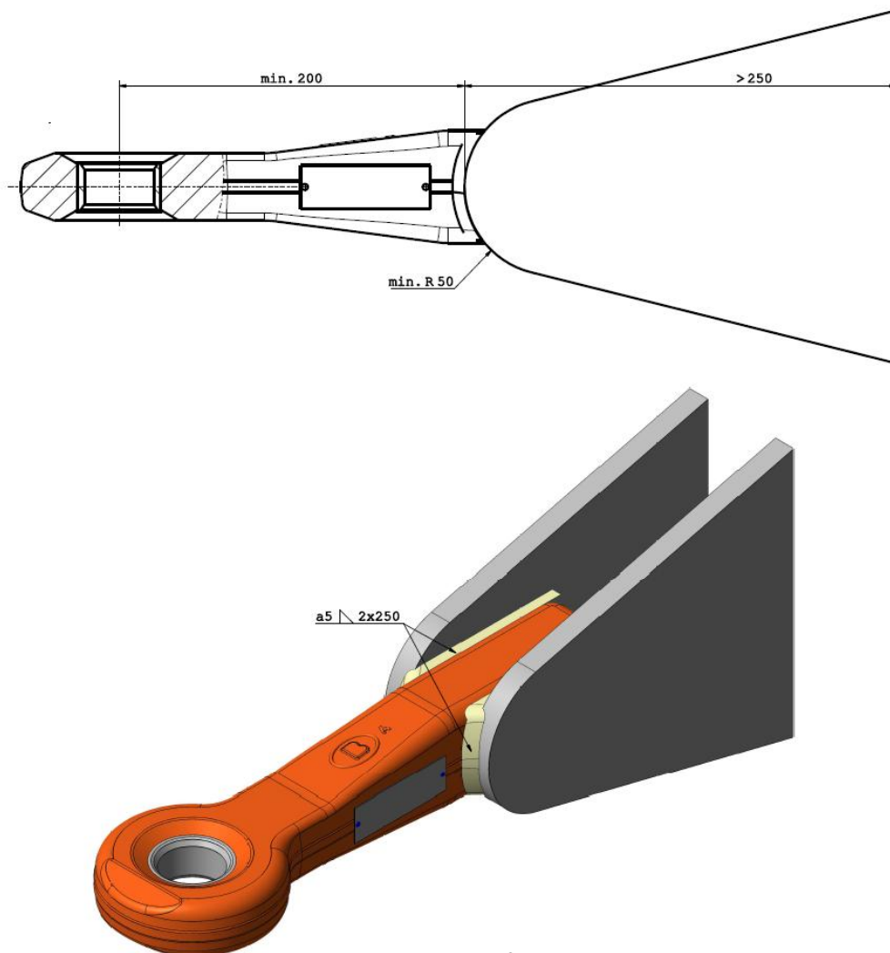
Abb. 1 Skizze Schweißverbindung
